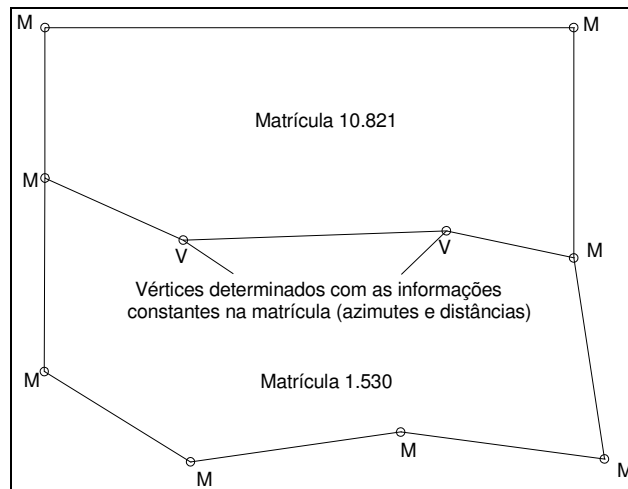
Figura 4 – Vértice tipo V, projetado
