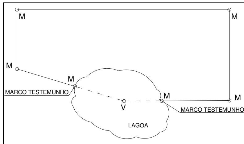
Figura 3 – Vértice tipo V, por determinação analítica
